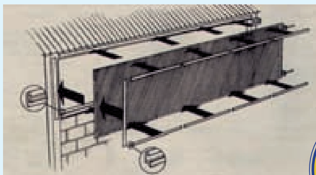
(Fest installierte Windschutznetze sind über spezielle Aluminiumprofile leicht an Gebäuden zu befestigen)
